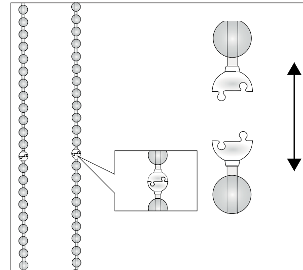
Dispositif de sécurité enfant par séparation de la chaînette de manoeuvre.
